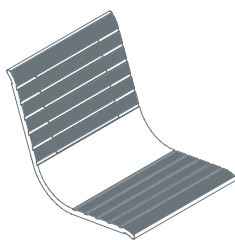
Wooden slats shell 1RS5521: L 52 D 65 H 48
