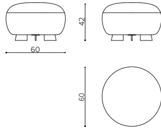
CD 60RO small round module modulo circolare piccolo petit module circulaire
