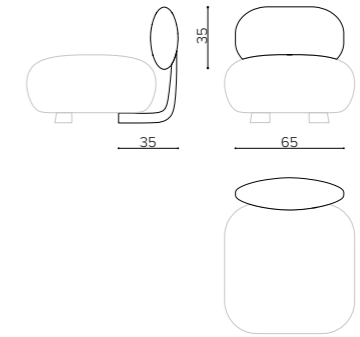
CD 75BR 75cm backrest module module for all large versions modulo schienale 75cm per tutte le versioni grandi module dossier 75cm pour toutes les grandes versions
