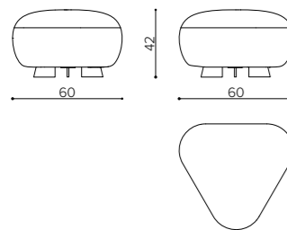
CD 60TR small triangular module modulo triangolare piccolo petit module triangulaire
