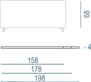
Akoestisch gestoffeerd bureauscherm tbv 122 cm hoog
