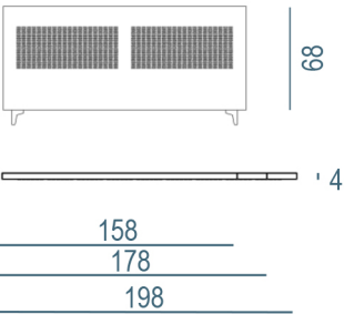
Akoestische bureauscherm met perforatie Sound and Vision 2.0 series
